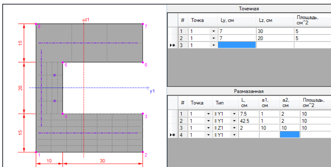
Рис. А.12. Пример задания арматуры для швеллера в Редакторе сечений/жесткостей
