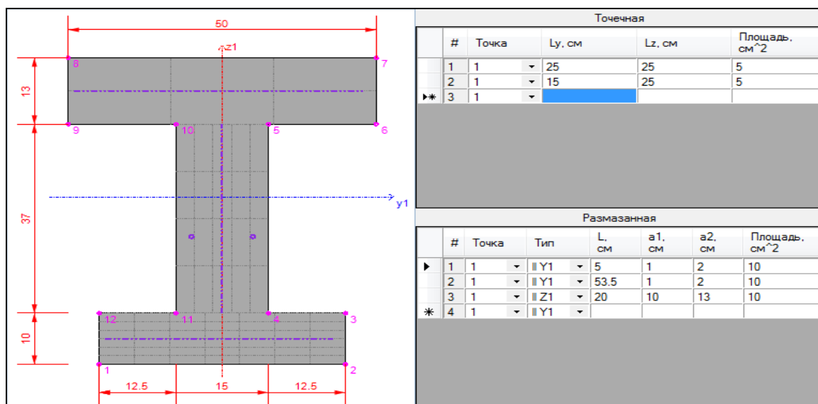
Рис. А.11. Пример задания арматуры для двутавра в Редакторе сечений/жесткостей
