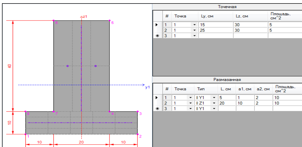
Рис. А.9. Пример задания арматуры для симметричного тавра (полка снизу) в Редакторе сечений/жесткостей
