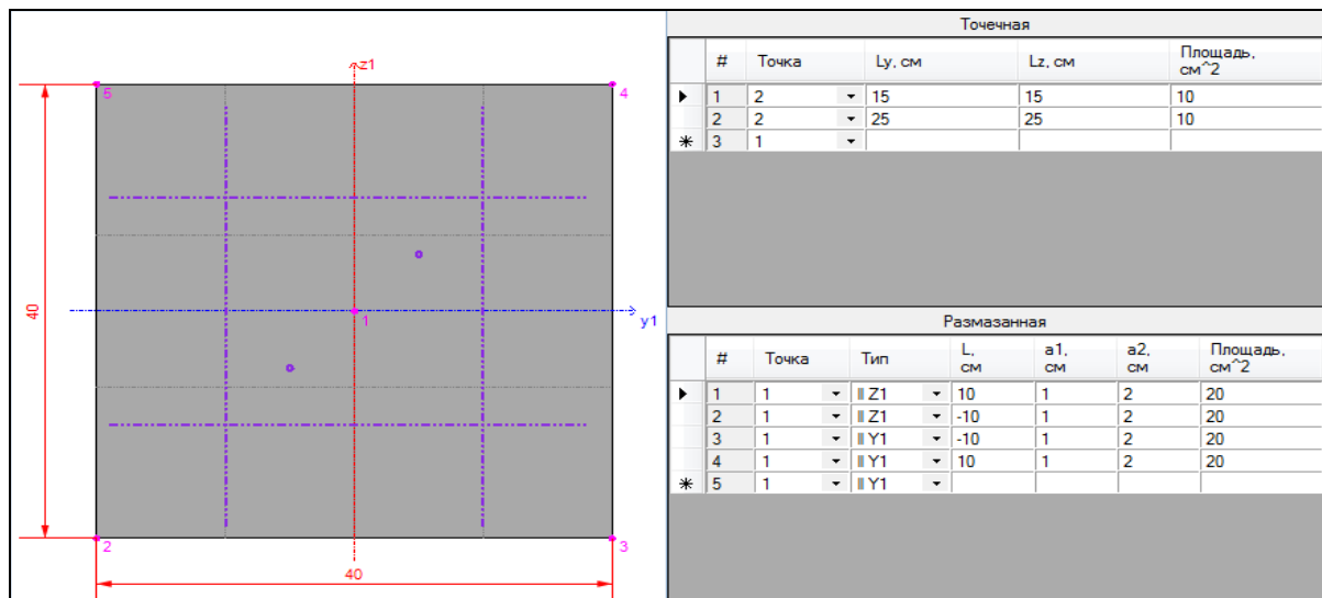
Рис. А.8. Пример задания арматуры для бруса в Редакторе сечений/жесткостей
