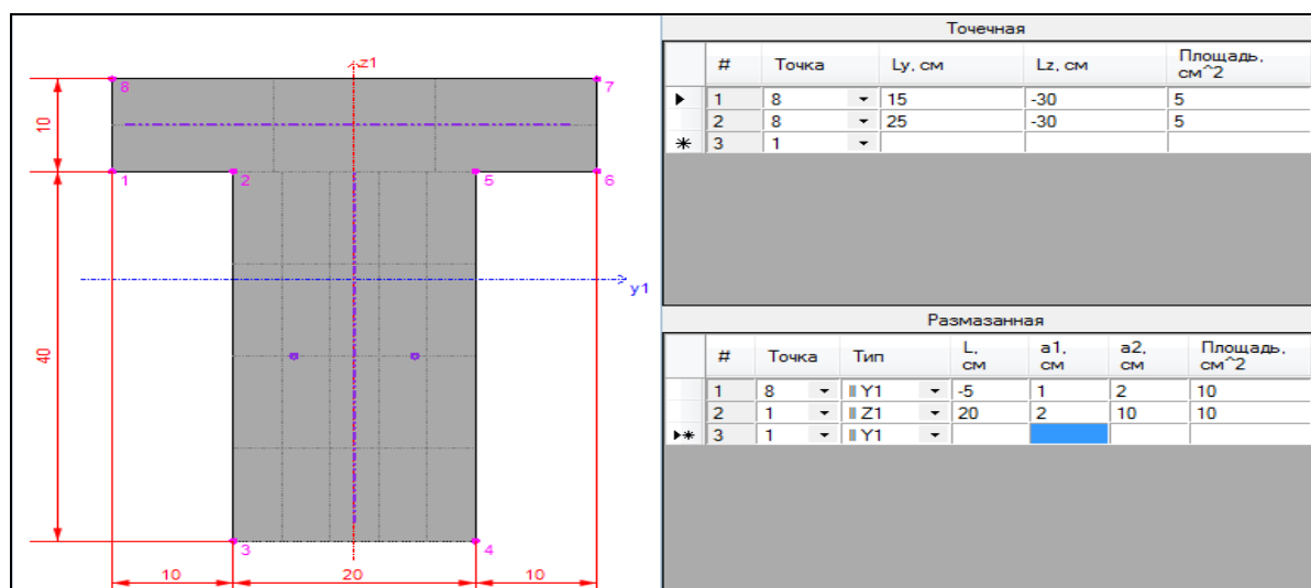
Рис. А.10. Пример задания арматуры для симметричного тавра (полка сверху) в Редакторе сечений/жесткостей
