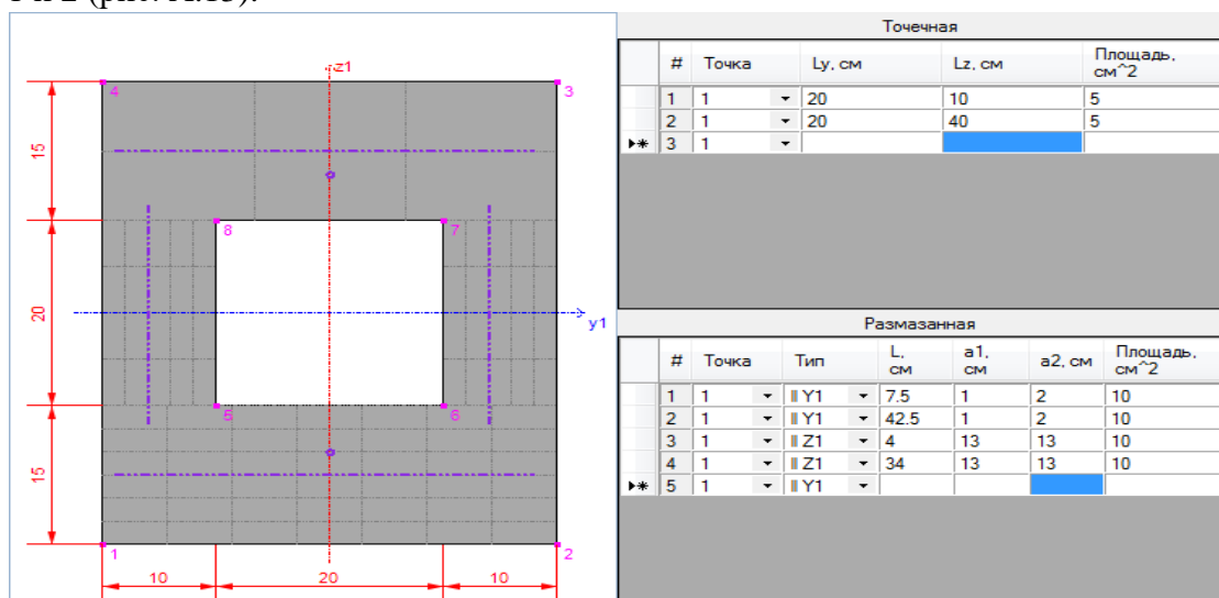
Рис. А.13. Пример задания арматуры для коробки в Редакторе сечений/жесткостей
